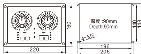
开孔尺寸 Hole dimension
